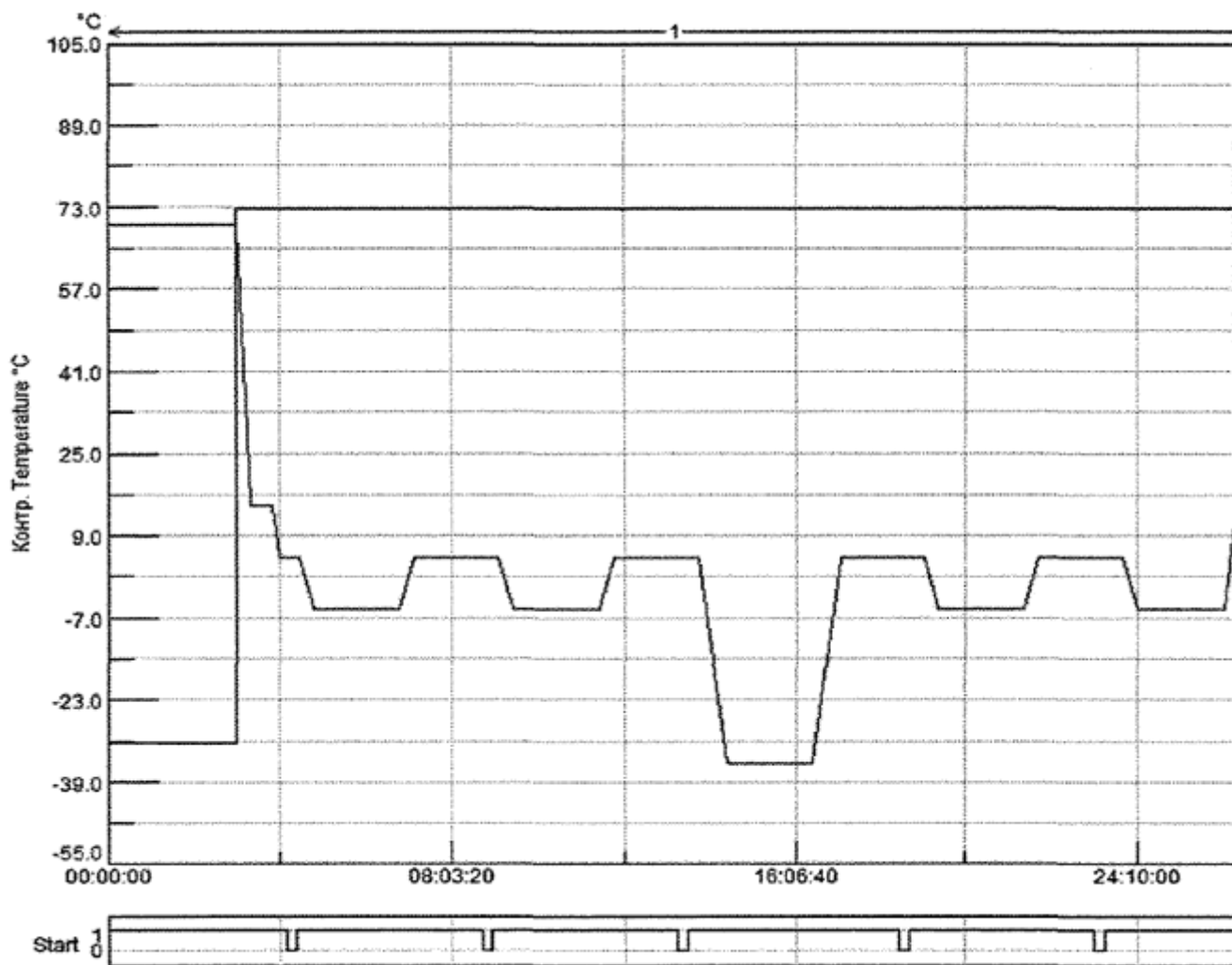
Рисунок А.1 - Графическая модель одного цикла климатических испытаний
