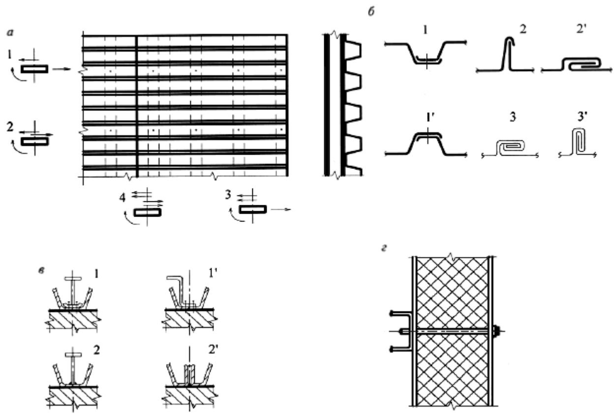
a - фрагмент конструкции покрытия со стальным профилированным настилом и схема действия сил на опорах (1 - соединения в среднем участке; 2 и 3 - соединения соответственно по продольным и поперечным полкам; 4 - соединения в месте пересечения продольных и поперечных полок); б - схема соединений по продольным полкам (1 и 1' - при расположении полок внахлест в нижнем и верхнем положениях соответственно для утепленных и холодных покрытий; 2 и 2' - простой стоячий и лежащий фальцы; 3 и 3' - двойной фальц, стоячий и лежащий); в - сдвигоустойчивые элементы (1 и 1' - на высокопрочных дюбелях; 2 - на контактной сварке; 2' - на дуговой сварке); г - фрагмент трехслойной стеновой панели на самосверлящем винте
