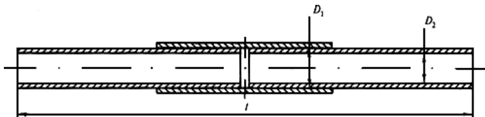
Рисунок 8 - Допускное соединение
