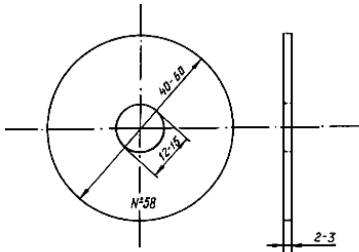
Рис.1. Индикатор внутренней коррозии
