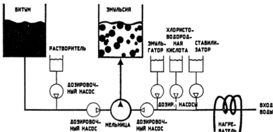
Рисунок 2 - Эмульсионная установка непрерывного действия
