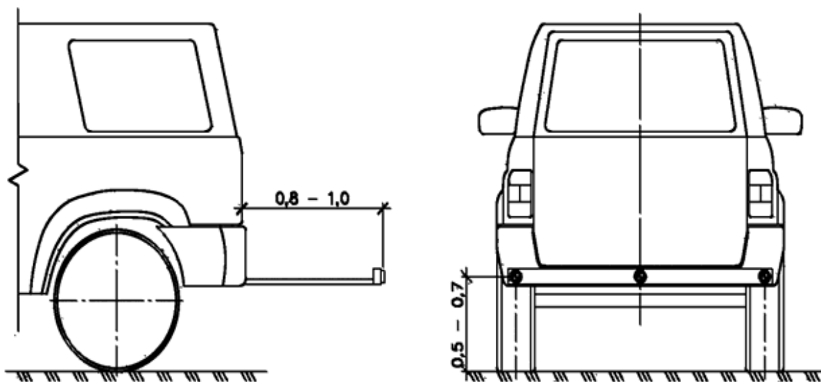
Рисунок Д.1 - Схема установки фильтров на автомобиль-лабораторию
