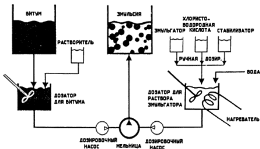
Рисунок 1 - Эмульсионная установка периодического действия
